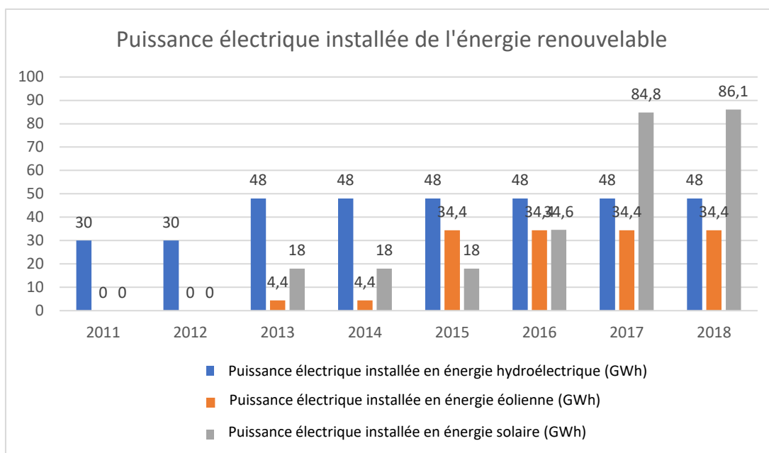
Graphique 8. Capacité électrique installée pour les sources renouvelables. Élaboration ad hoc. Source : Banque Africaine de Développement
